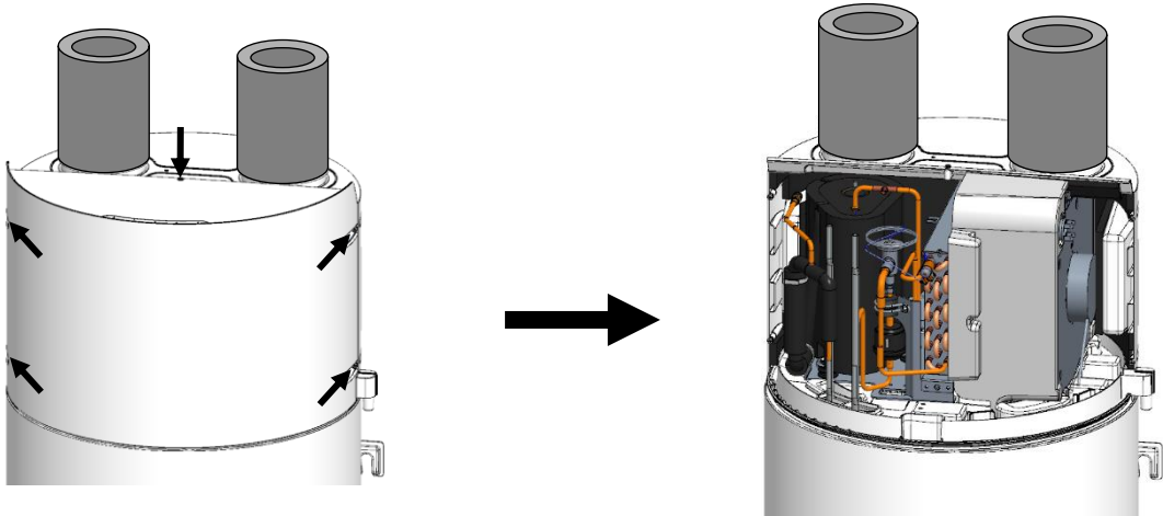
Desatornille la tapa frontal (x 5 tornillos)
