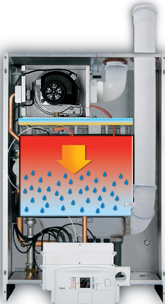
Fenómeno de la Combustión/Condensación
