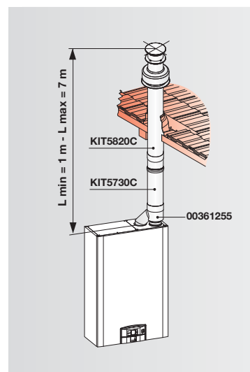
CONDUCTOS COAXIALES Ø 80/125 mm Tipo C33
