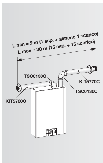
CONDUCTOS SEPARADOS Ø 80 Tipo C53
