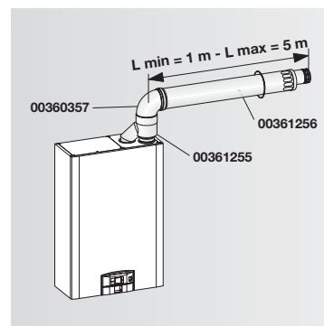
CONDUCTOS COAXIALES Ø 80/125 mm Tipo C13
